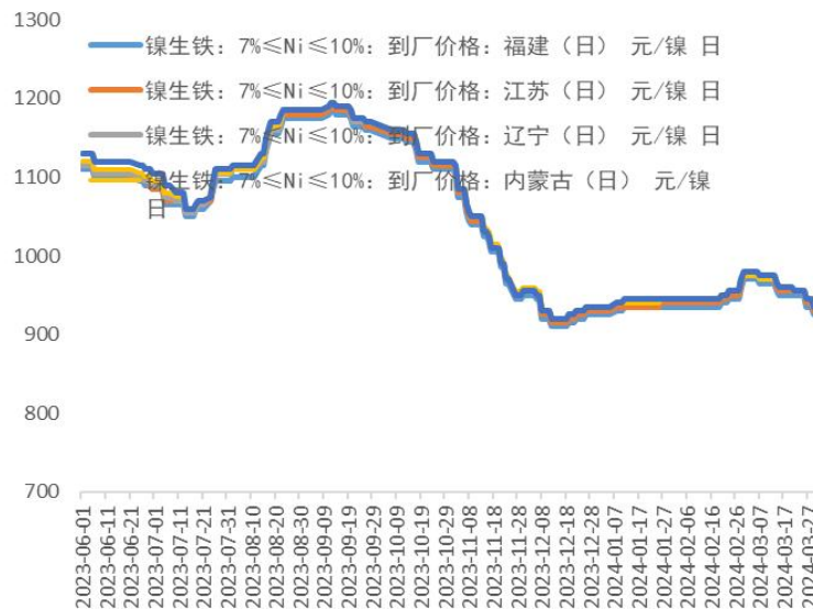
图2 镍生铁价格走势
