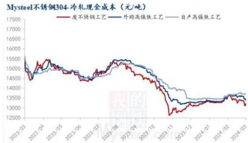
图16 不锈钢生产成本
