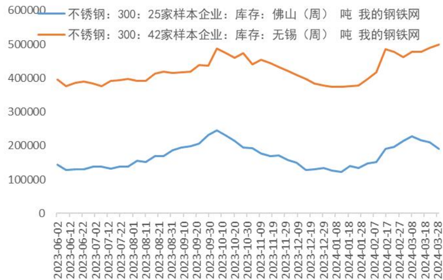
图11 300系不锈钢社会库存：佛山、无锡
